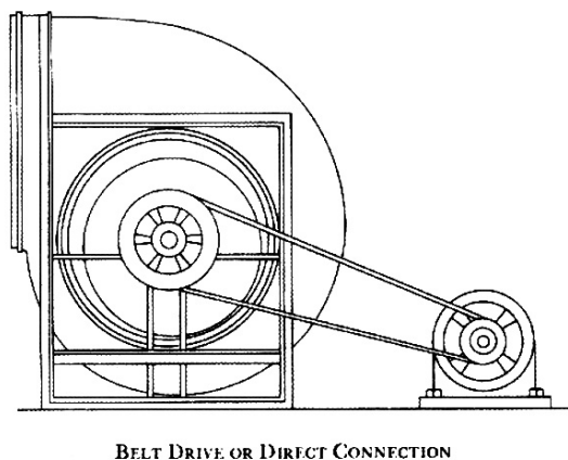
Fig. 1 – Centrifugal Fan
