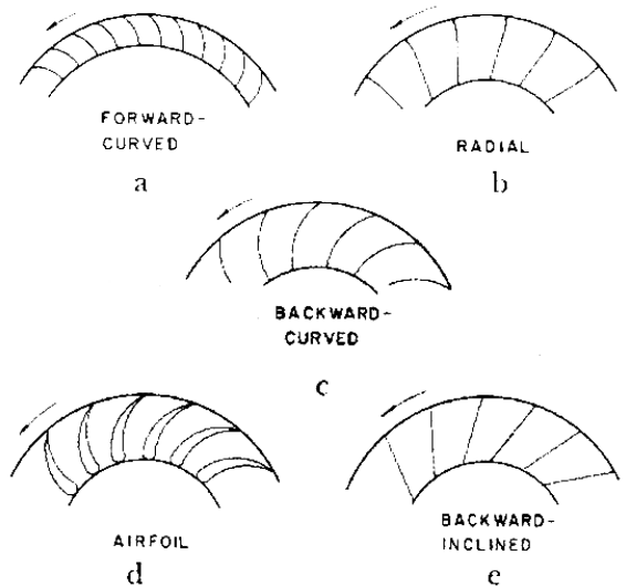
Fig. 5 – Fan Blades
